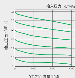
YT-220 流量 (LPM)
