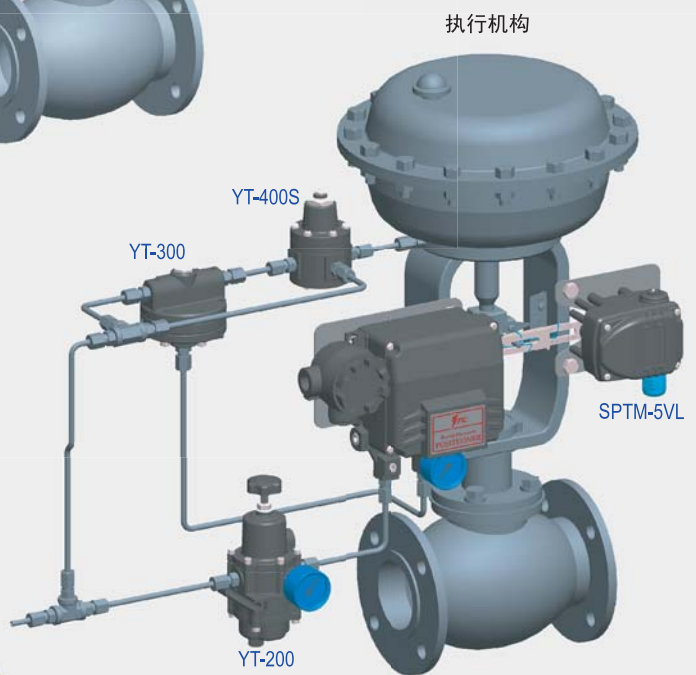
YT-1000L 单作用安装例图
