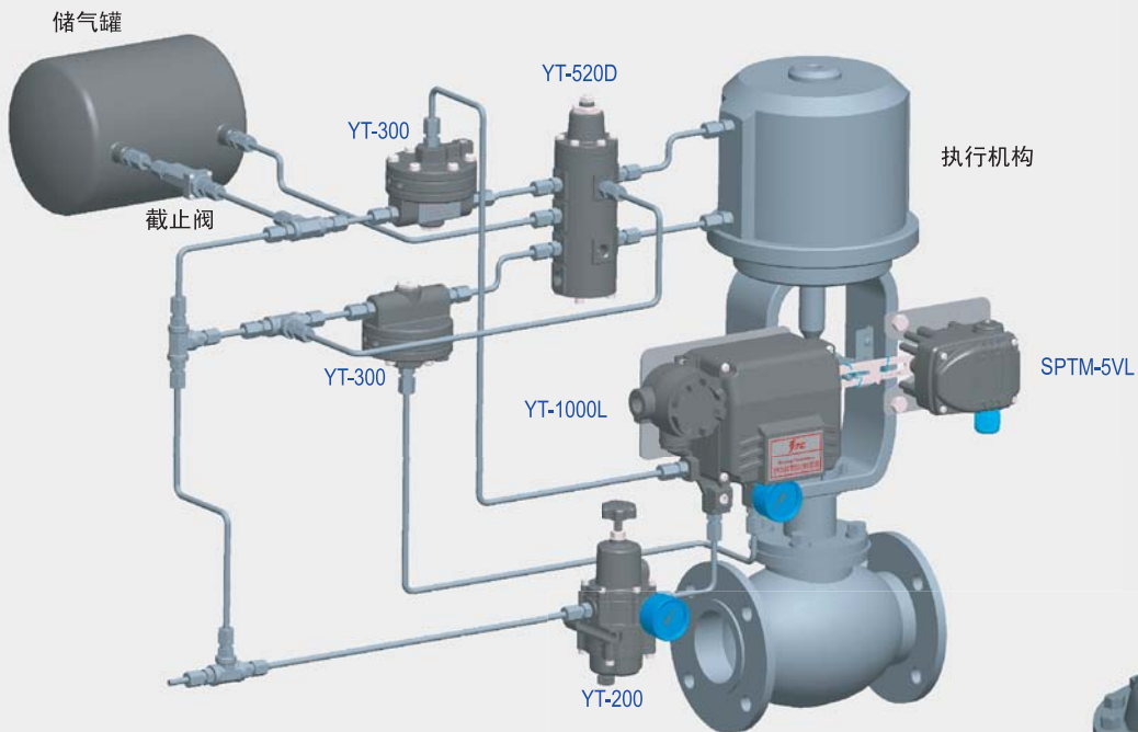
YT-1000L 双作用安装例图
