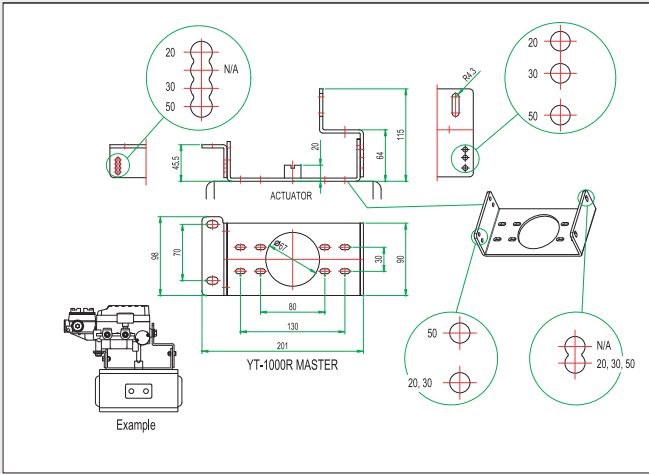
YT-1000R 系列支架
