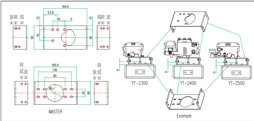
YT-2300R & YT-2400R & YT-2500R & YT-2550 & YT-2600 & 3400 系列支架
