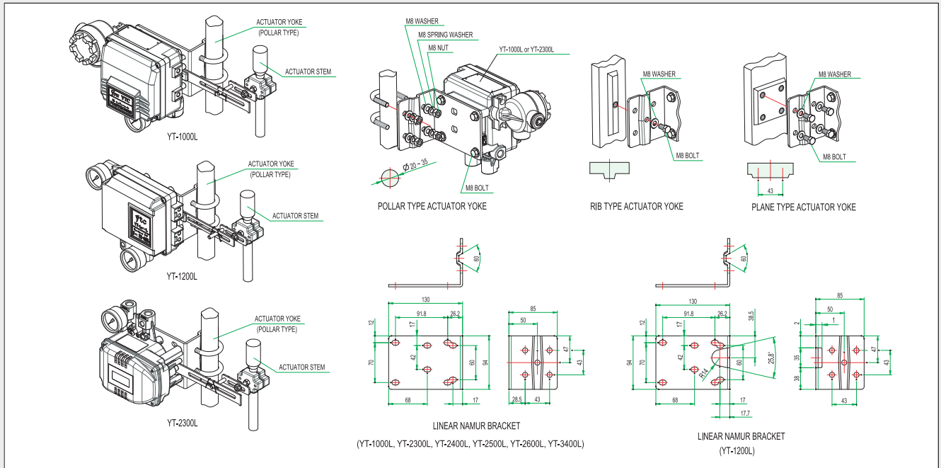
YT-1000L & 1200L & 2300L Namur 系列支架
