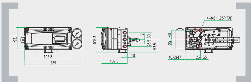
YT-3300 + 限位开关
