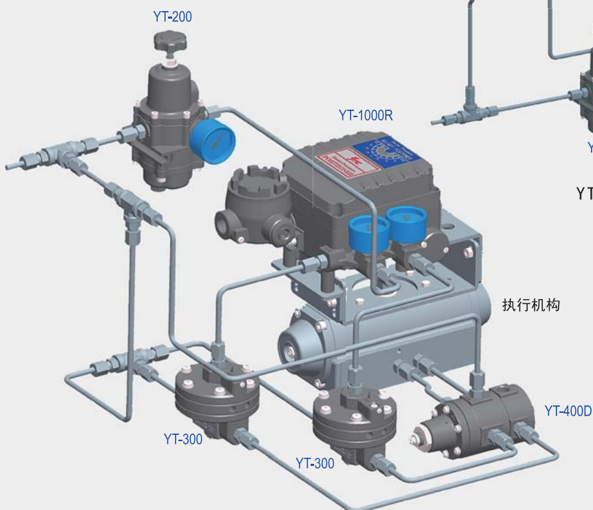
YT-1000R 双作用安装例图
