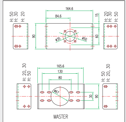
YT-3300 系列支架
