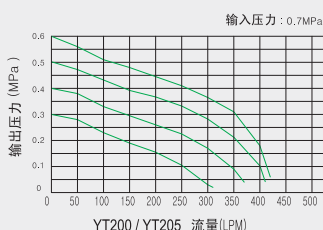
YT200 / YT205 流量 (LPM)
