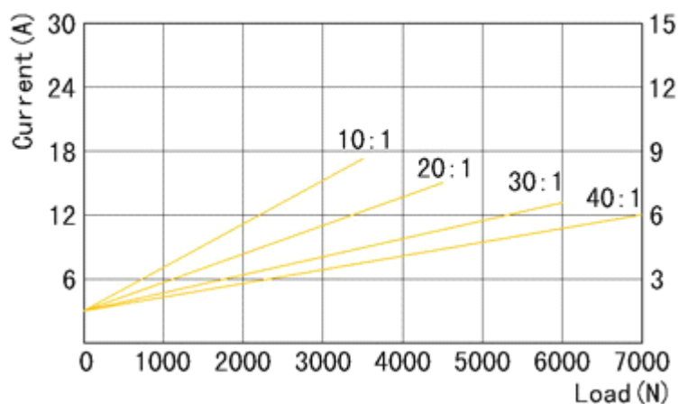
12V DC 电流与负载关系图 24V DC Current vs load
