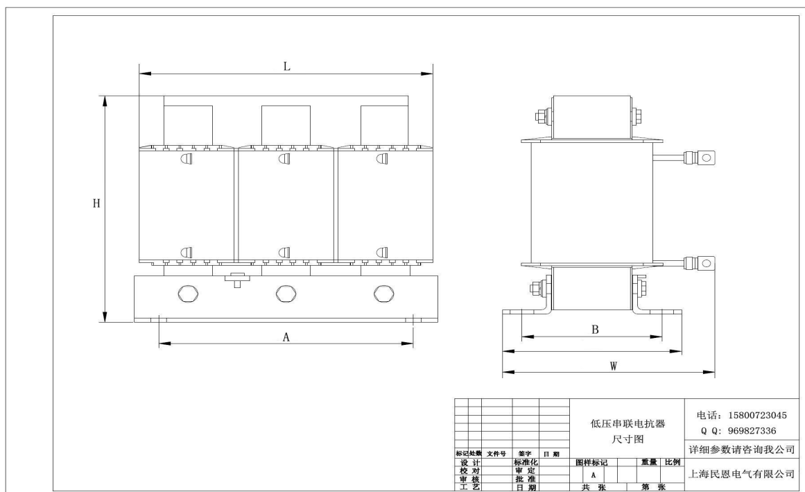
CKSG-2.1/0.45-7 低压串联电抗器尺寸图：
