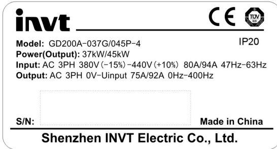
图 3-3 产品铭牌
