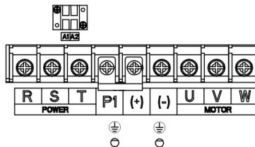
图 4-11 37~55kW 主回路端子示意图
