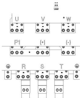
图 4-15 350~500kW 主回路端示意图
