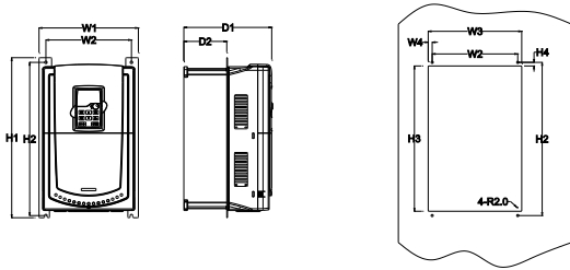
18.5-30kW 法兰安装示意图
