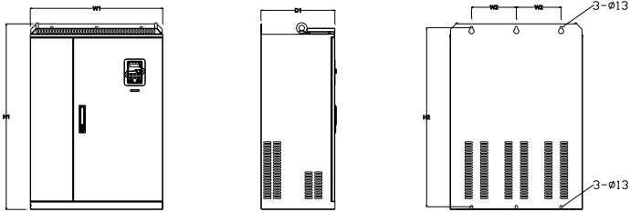
220-315kW 壁挂安装示意图
