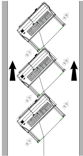
图 4-5 倾斜安装
