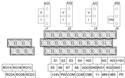
图 4-19 15kW（含）以下控制端子示意图
