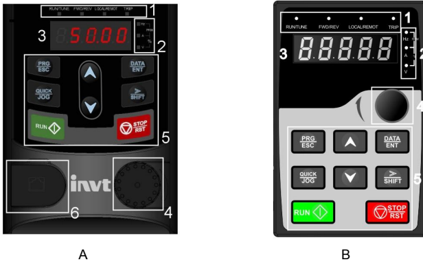
图 5-1 键盘示意图
