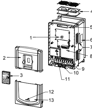
图 3-4 产品结构示意图
