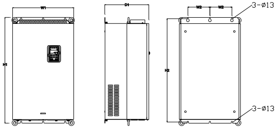
132-200kW 壁挂安装示意图
