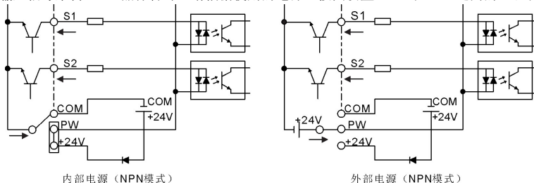
图 4-22 NPN 模式示意图
