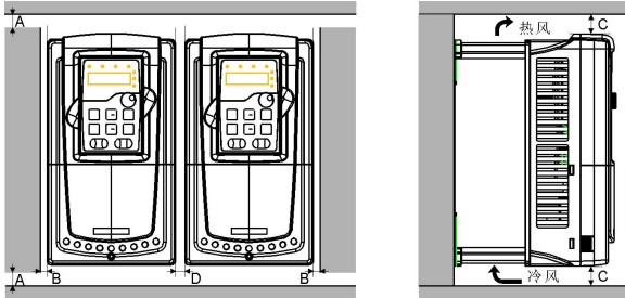
图 4-3 并行安装
