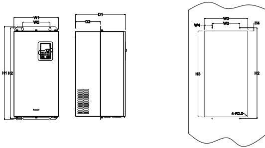
37-110kW 法兰安装示意图
