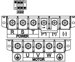
图 4-12 75~110kW 主回路端示意图
