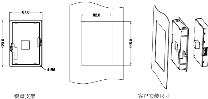
键盘支架
