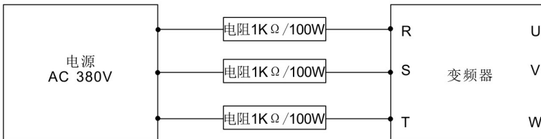
图 10-1 380V 驱动装置充电电路示例
