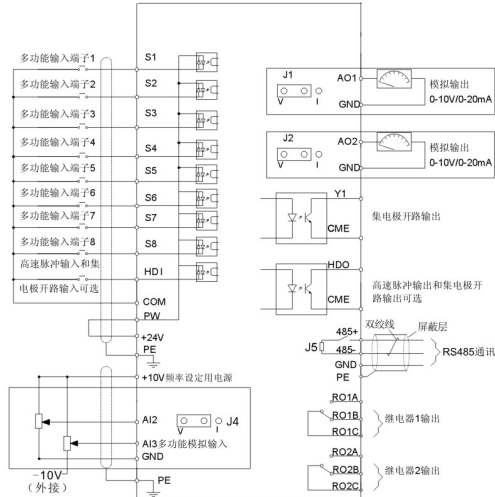
图 4-18 控制回路接线图
