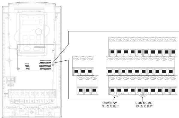
图 4-21 U 型短接位置示意图
