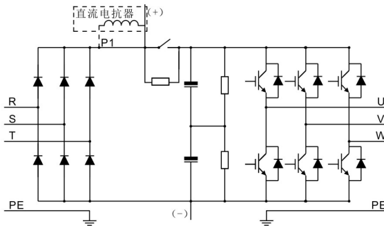
图 3-2 主回路简图（大于 37kW（含））
