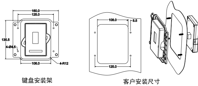
37~500kW 键盘安装架 (标配)
