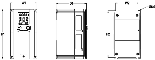
0.75-15kW 壁挂安装示意图
