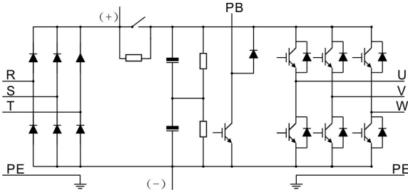
图 3-1 主回路简图（小于 30kW（含））
