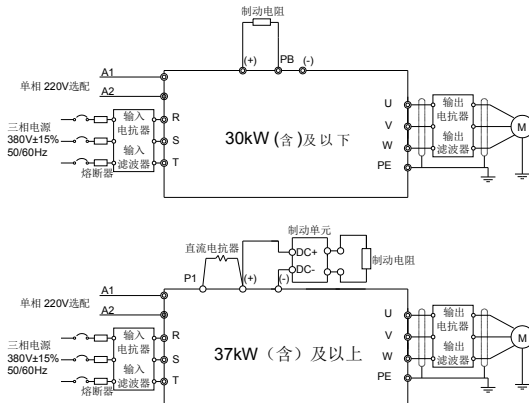
图 4-6 主回路接线图
