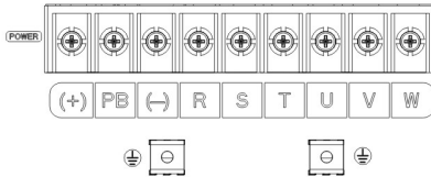
图 4-8 7.5~15kW 主回路端子示意图
