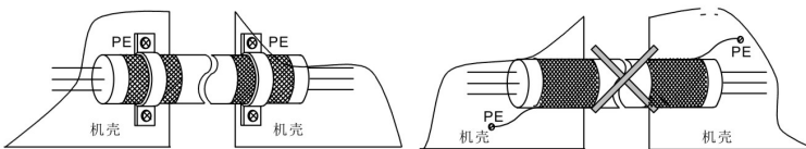
图 4-17 360 度环接示意图
