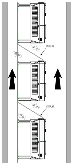
图 4-4 垂直安装
