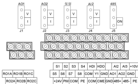
图 4-20 18.5kW（含）以上控制端子示意图
