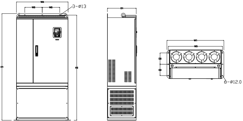
220-315kW 落地安装示意图
