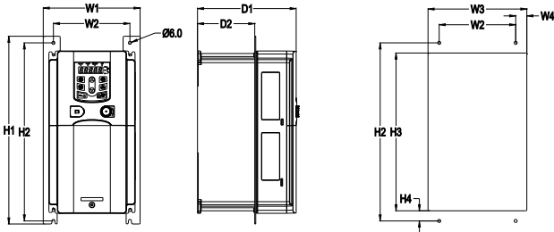
0.75-15kW 法兰安装示意图
