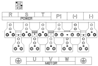
图 4-14 220~315kW 主回路端示意图
