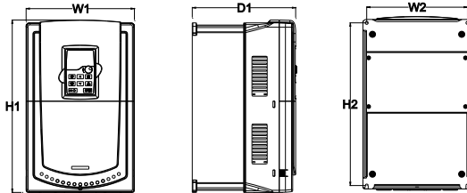
18.5-30kW 壁挂安装示意图
