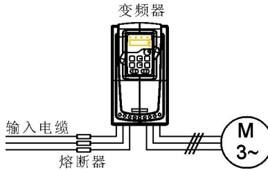
图 4-24 熔断器配置图
