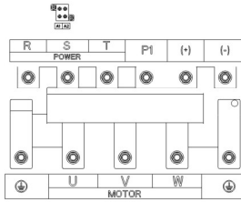
图 4-13 132~200kW 主回路端示意图
