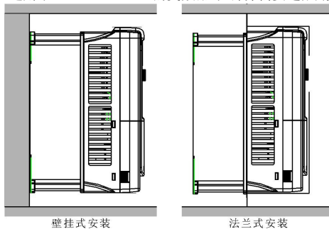
图 4-2 安装方式
