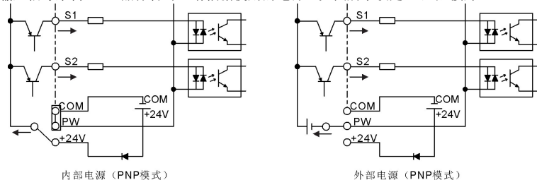
图 4-23 PNP 模式示意图
