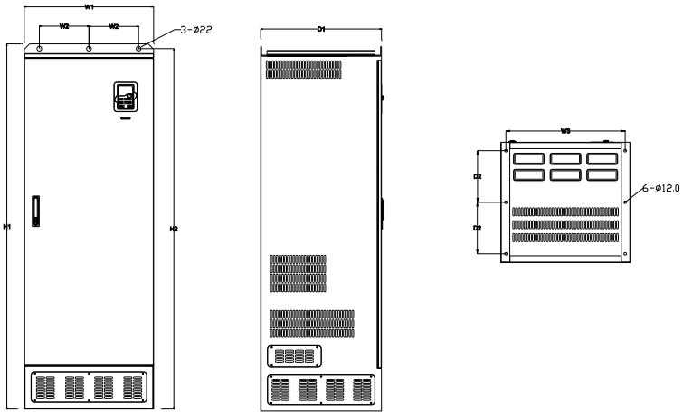
350-500kW 落地安装示意图
