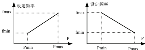
(1)正作用特性
