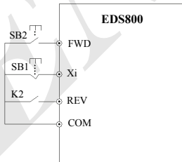
图 6-33 三线式运转模式 2
