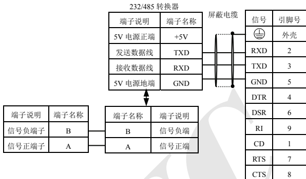
图 3-12 485 通讯配线
