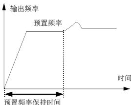
图 6-18 闭环预置频率运行示意图
