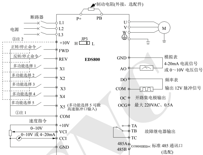
图 3-6 基本配线图
