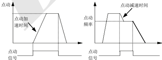
图 6-11 点动运行
