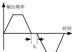
图 6-9 正反转死区时间
