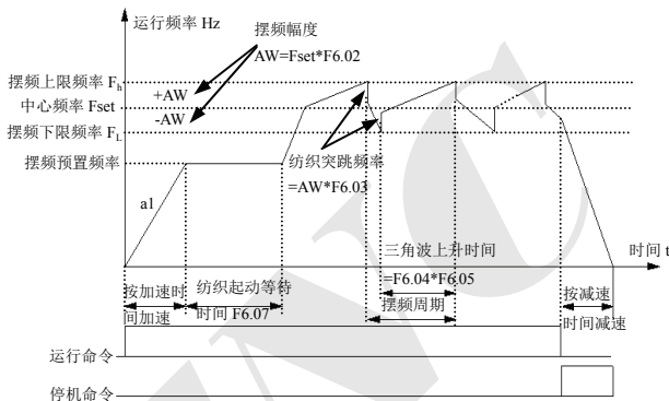
图 6-38 摆频示意图
