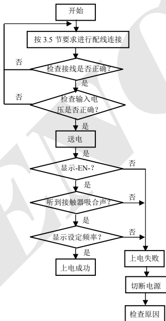
图 4-12 变频器初次上电操作流程
