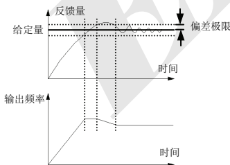
图 6-17 偏差极限示意图
