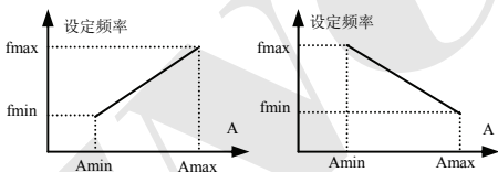
(1)正作用特性
