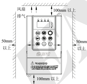
图 3-1 安装的间隔距离图
