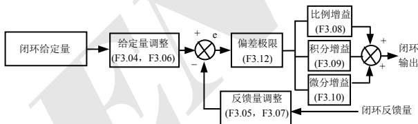
图 6-14 PID 控制原理框图
