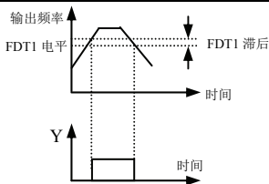
图 6-36 频率水平检测示意图
