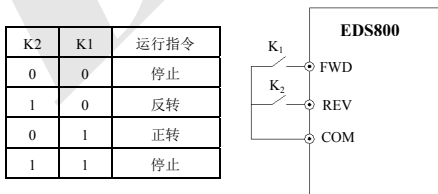
图 6-30 两线式运转模式 1
