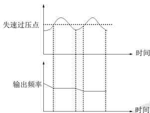
图 6-41 过压失速功能
