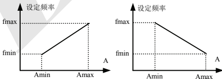
(1)正作用特性
