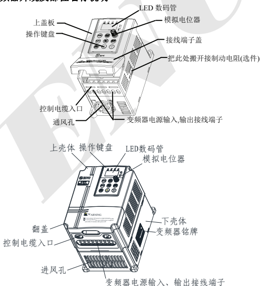
图 2-3 变频器各部位名称示意图
