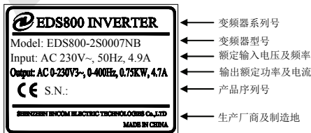
图 2-2 变频器铭牌
